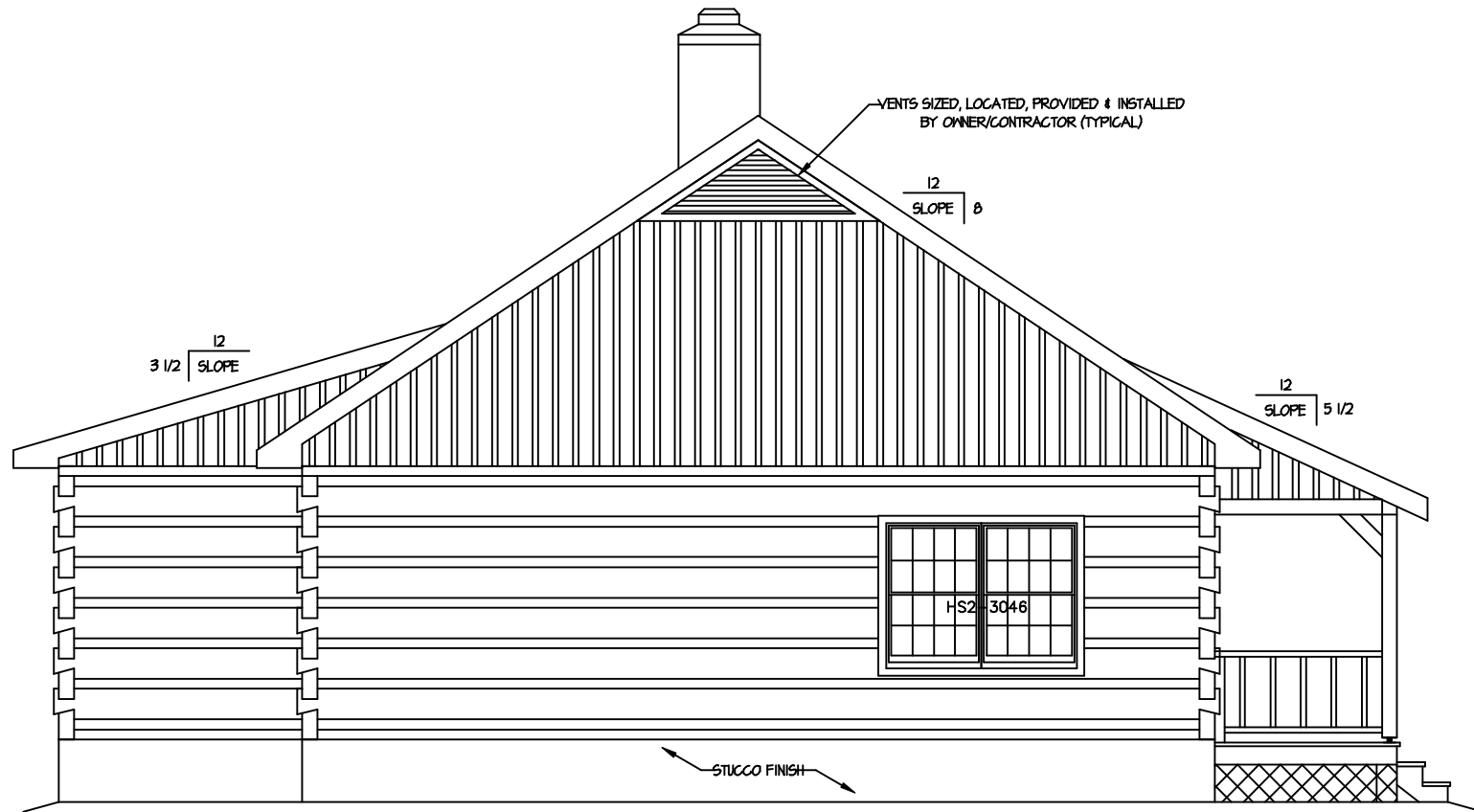
PLAN LEFT
