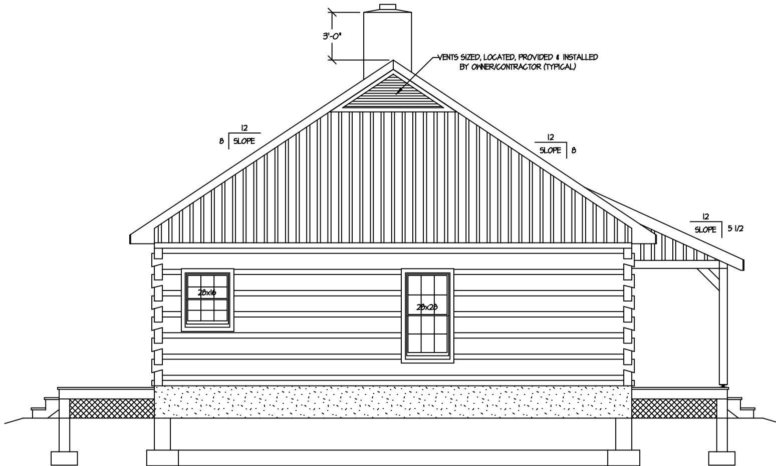
PLAN LEFT
